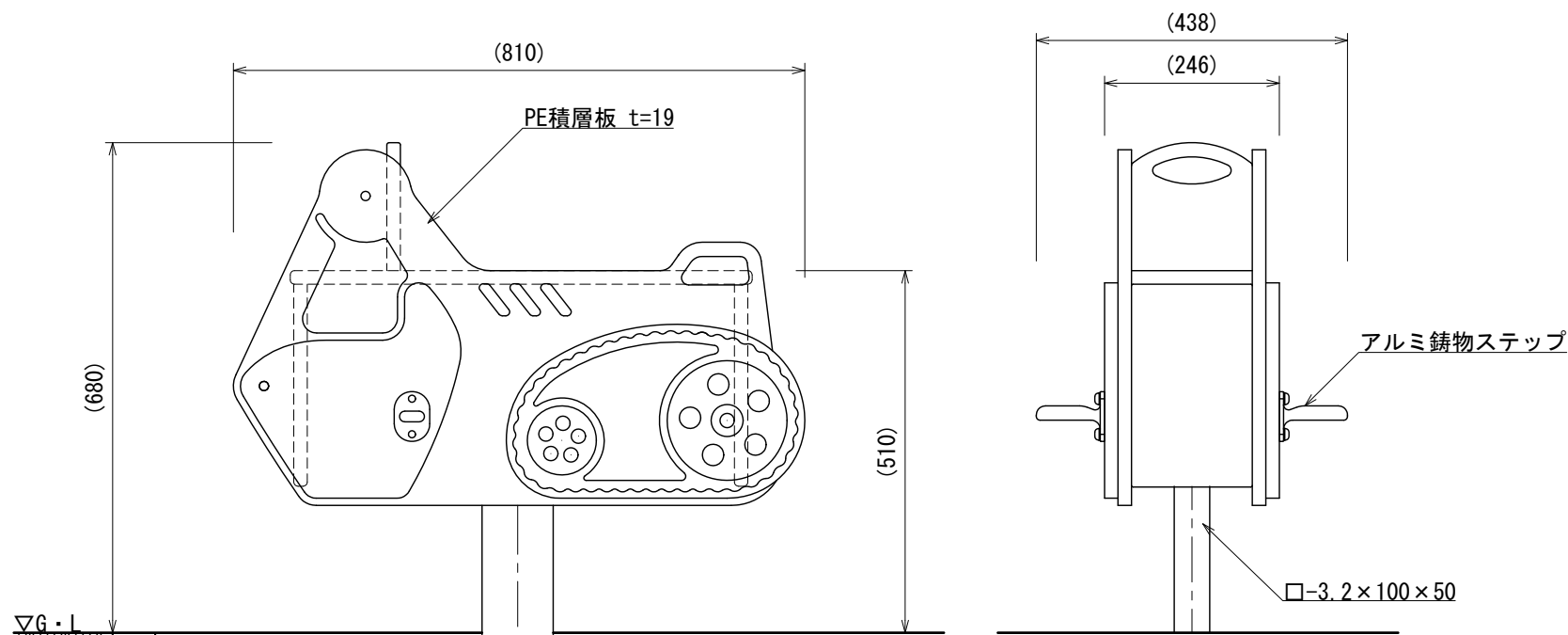
側面図
