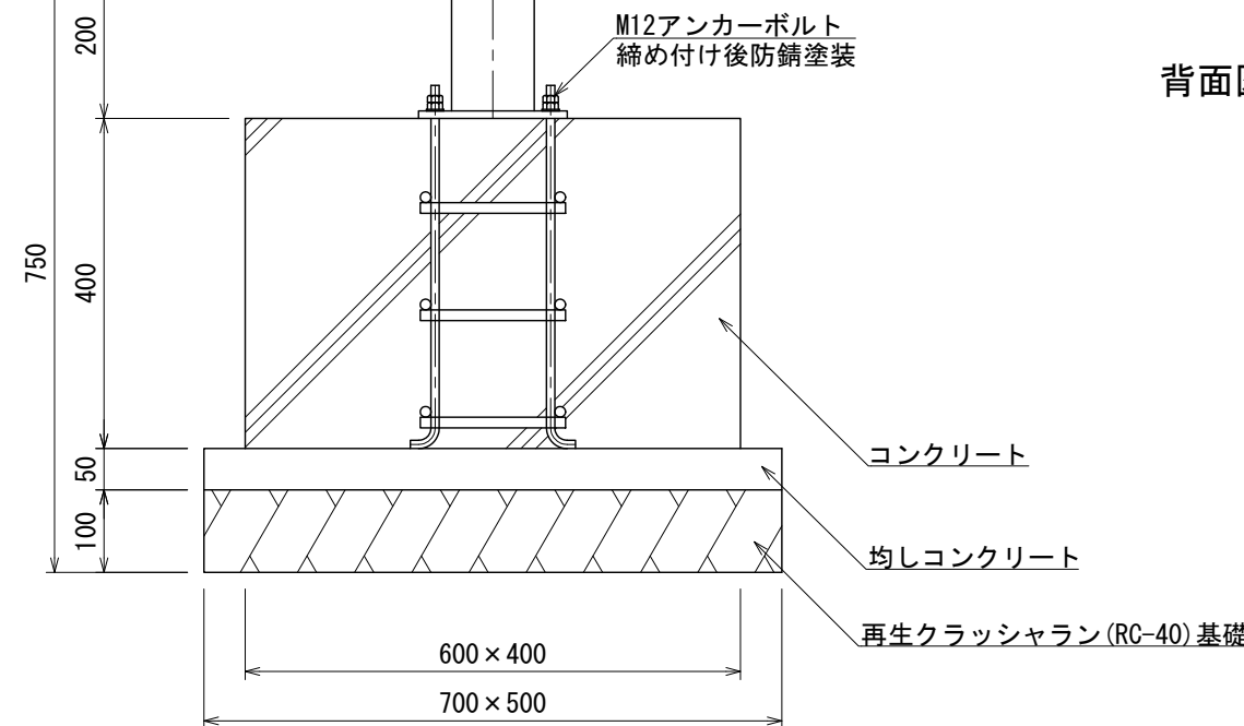
立面図
