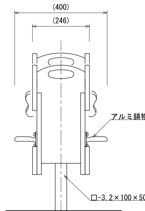
背面図
