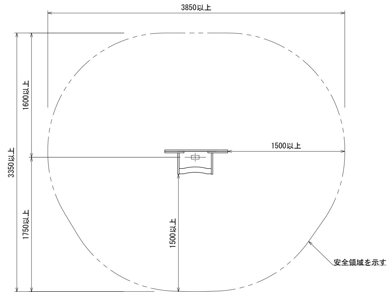
安全領域図 S=1:30
