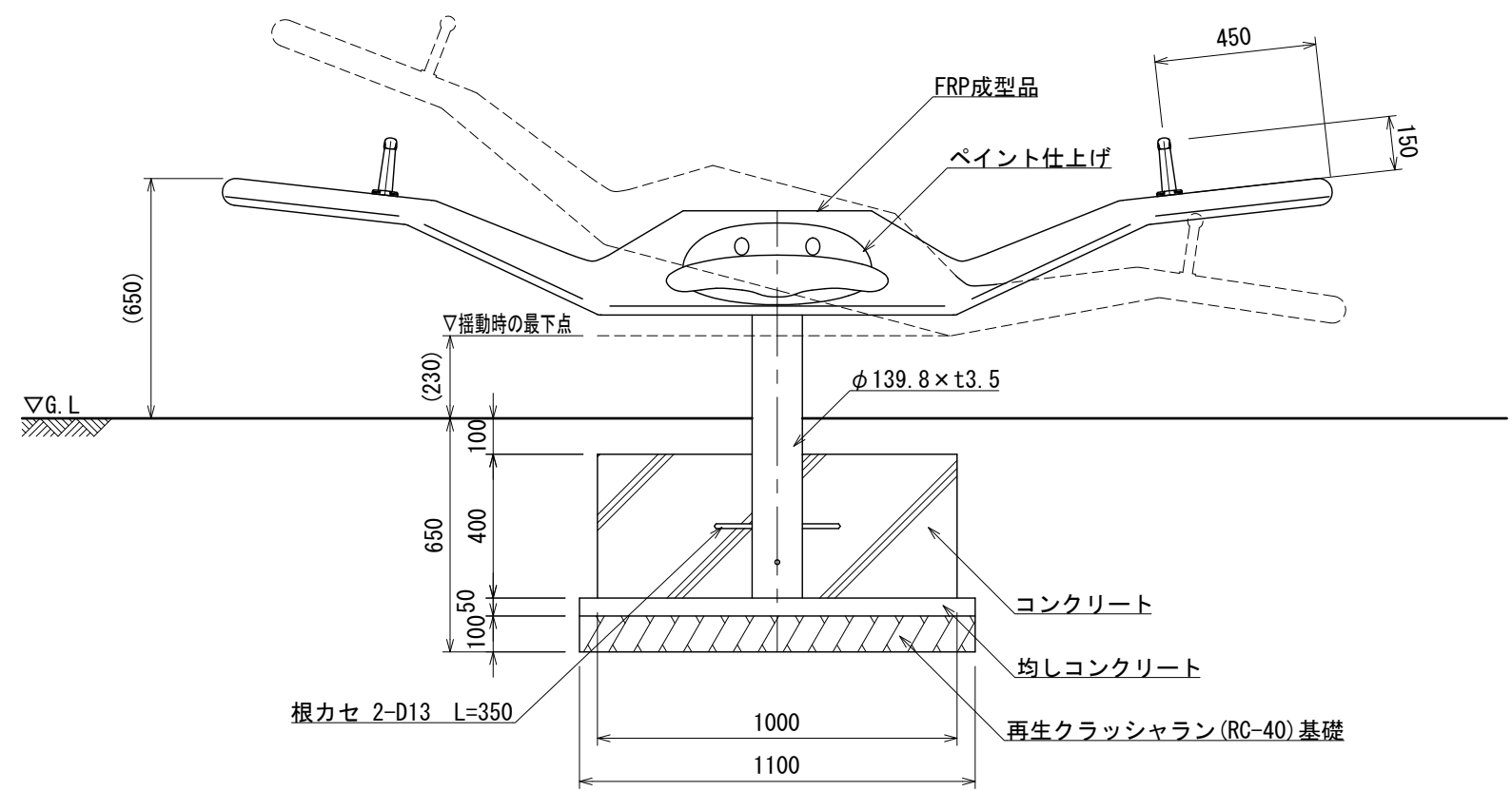
立面図
