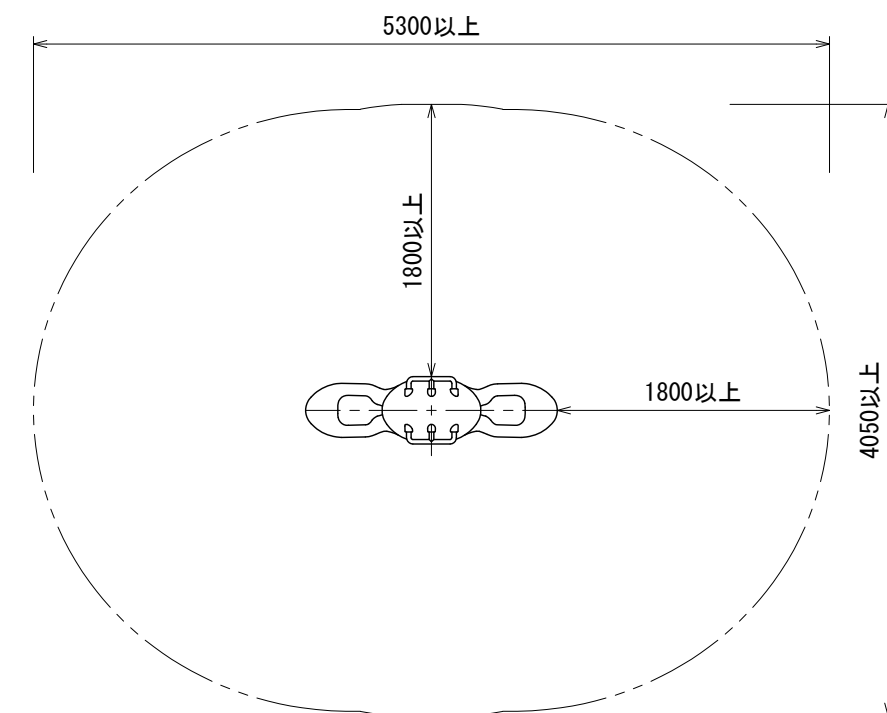
安全領域図 S=1:50
