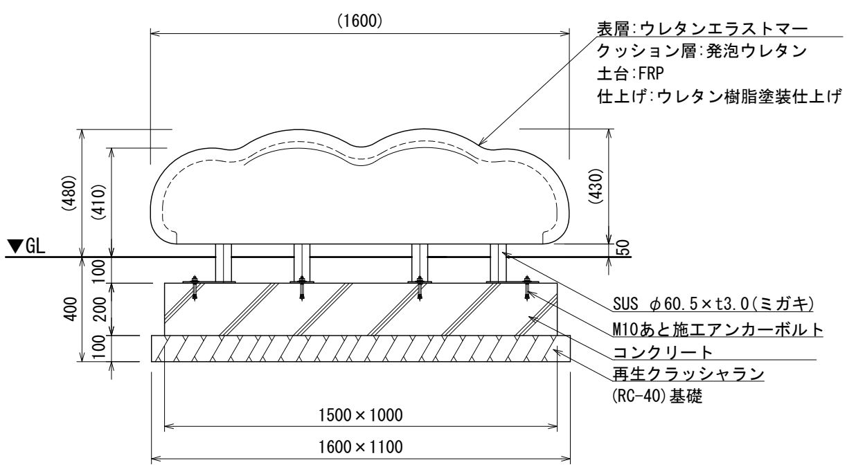
立面図
