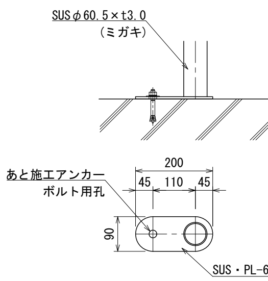
基礎固定部 S=1:10
