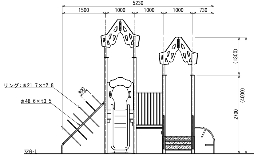
側面図
