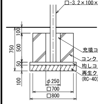
基礎詳細図 S=1:20 (A3 S=1:40)
