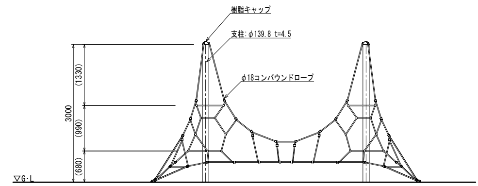
立面図
