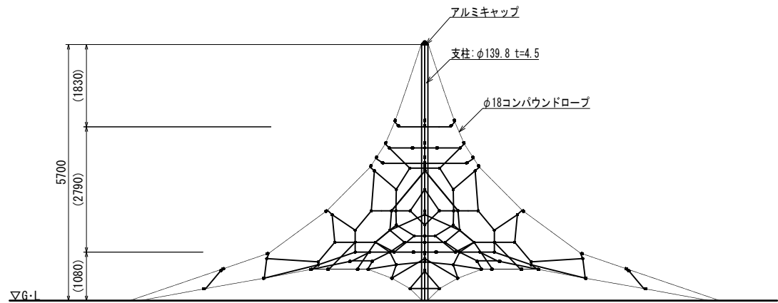
立面図
