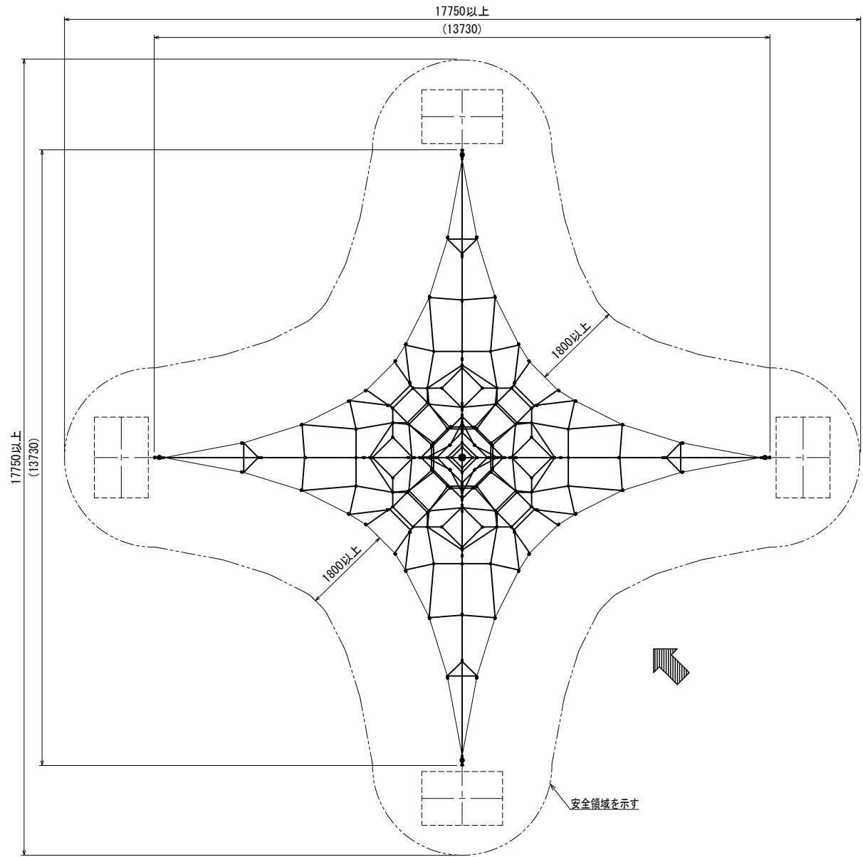
平面図
