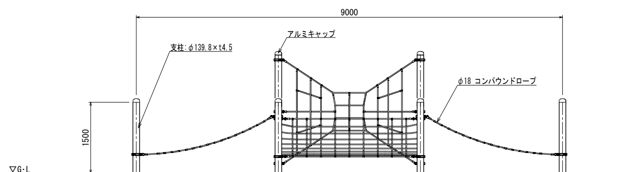
立面图
