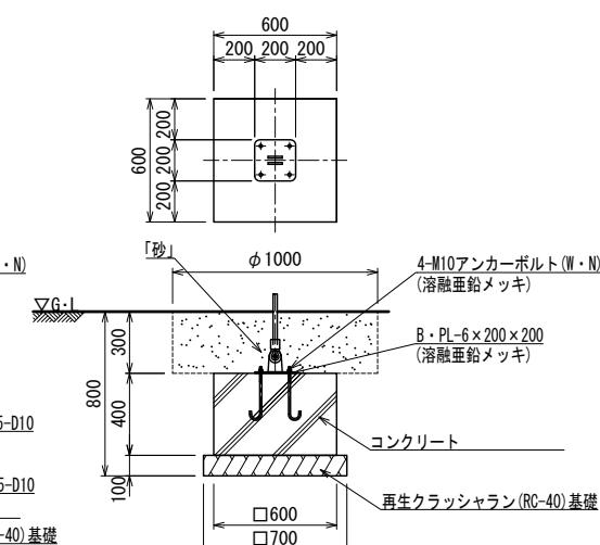
B基礎詳細図 S=1:20
