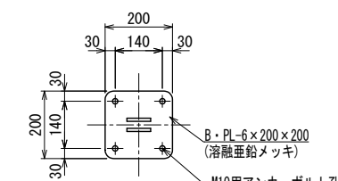
Bベースプレート詳細図 S=1:10
