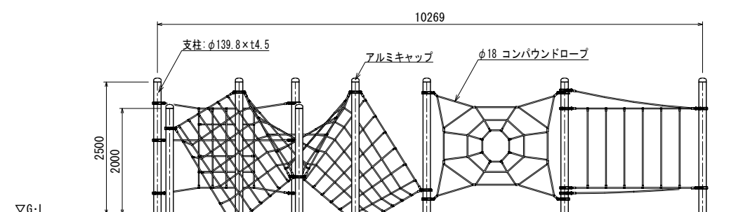
立面图
