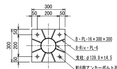
Aベースプレート詳細図 S=1:10
