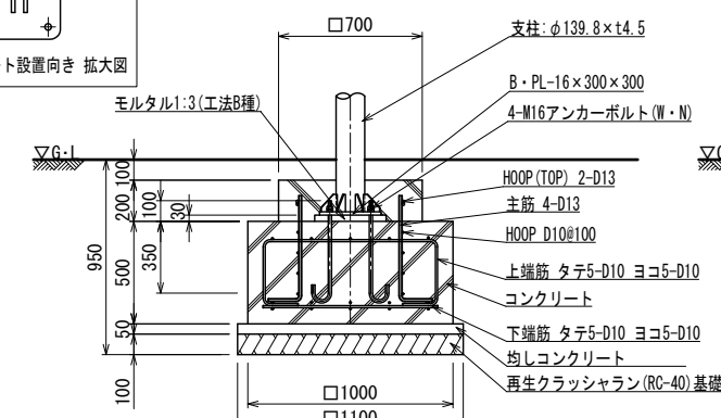
A基礎詳細図 S=1:20
