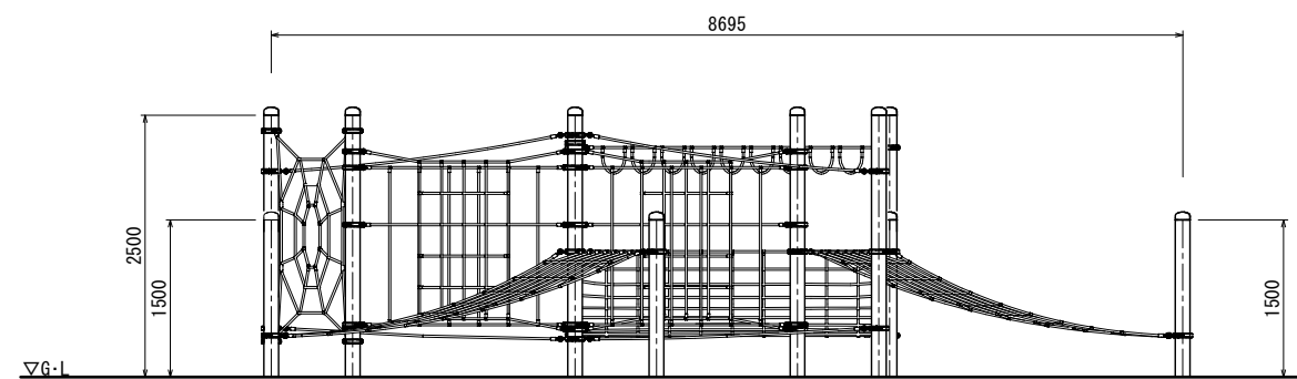
側面図
