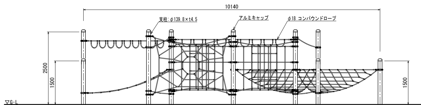
立面図
