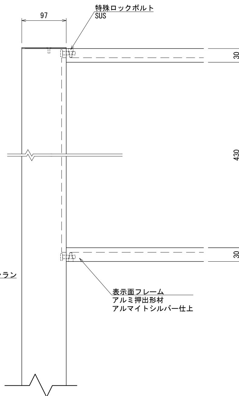
【正面図 S=1:5】
