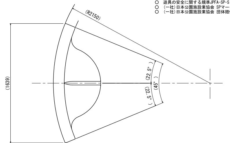
砂場枠標準断面図 S=1:15 (A1) S=1:30 (A3)
