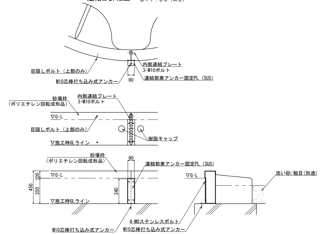
連結部詳細図 S=1:15 (A1) S=1:30 (A3)
