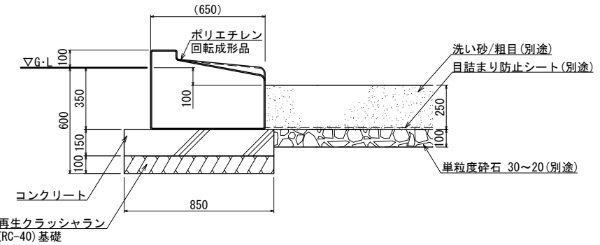
連結部詳細図 S=1:15 (A1) S=1:30 (A3)
