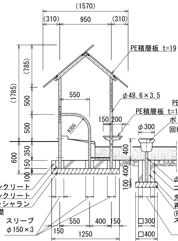
立面図
