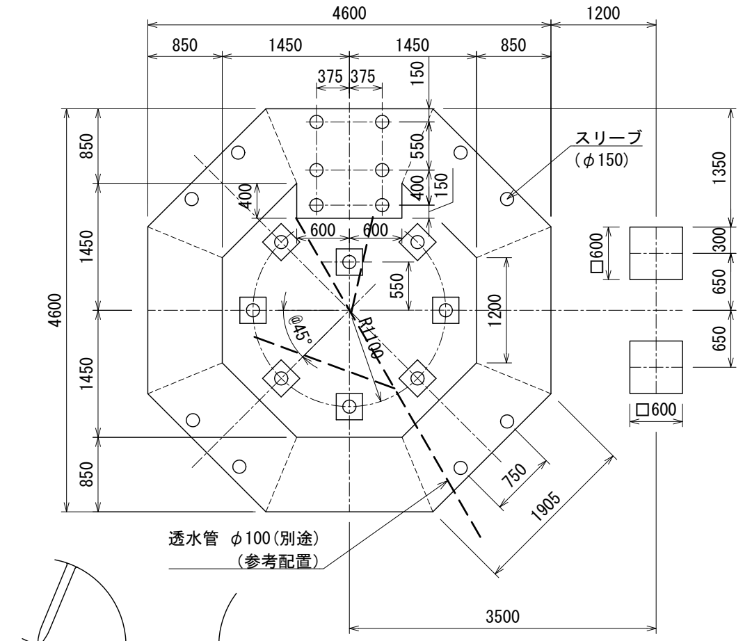
基礎伏図
