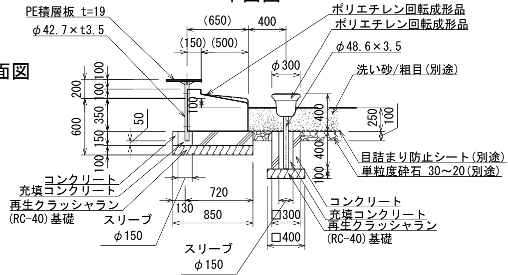
立面図
