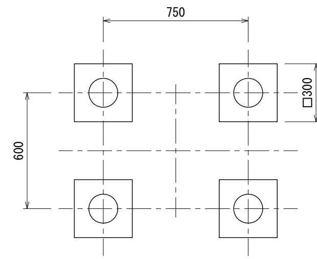
基礎伏図
