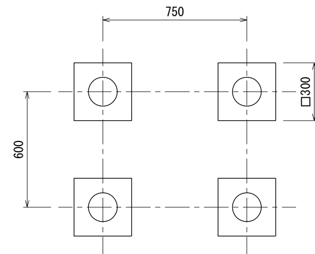
基礎伏図
