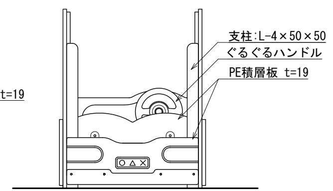
背面
