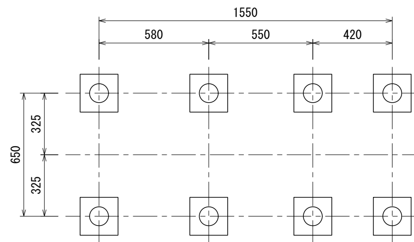
基礎伏図
