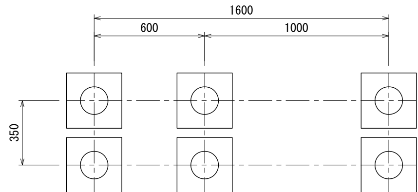
基礎伏図
