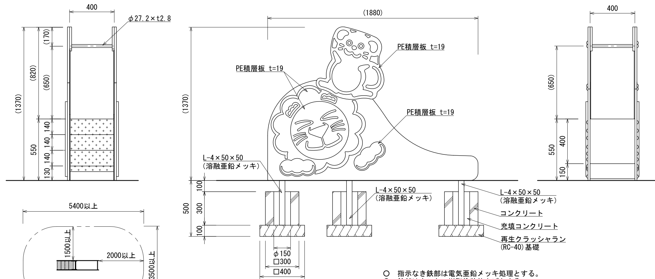
基礎伏図
