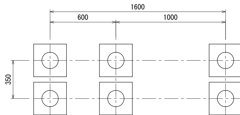
基礎伏図
