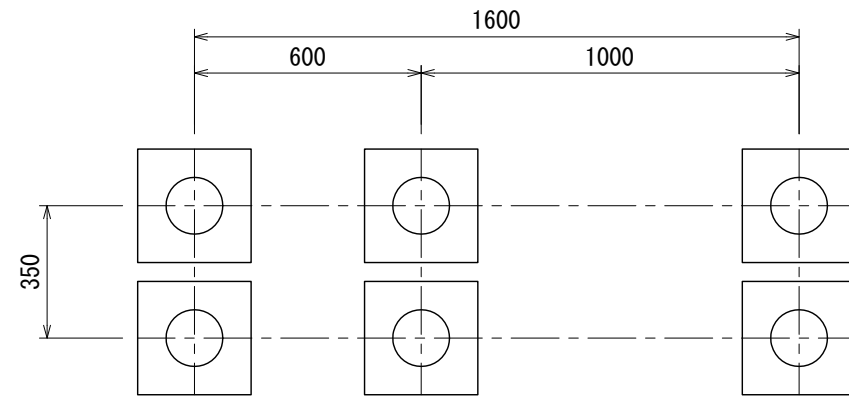
基礎伏図
