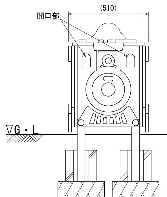
正面図
