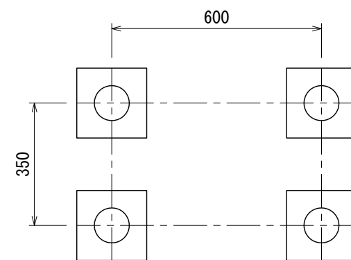
基礎伏図
