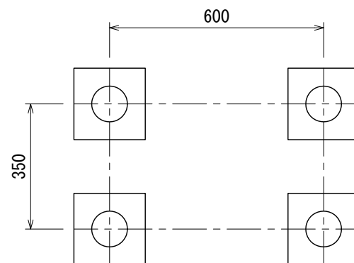
基礎伏図
