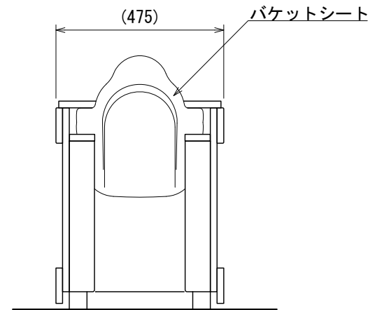
背面図
