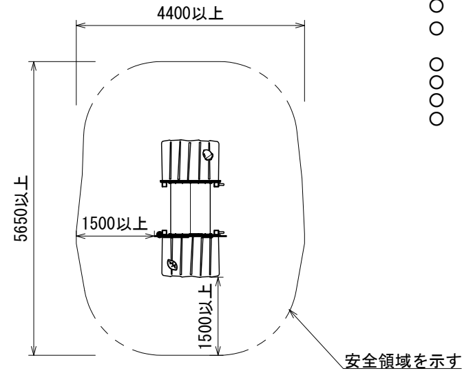
安全領域図 S=1:100
