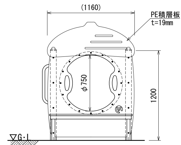
背面図
