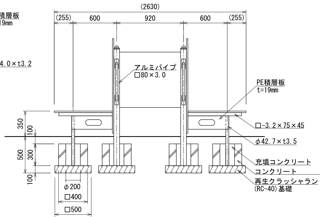
側面図
