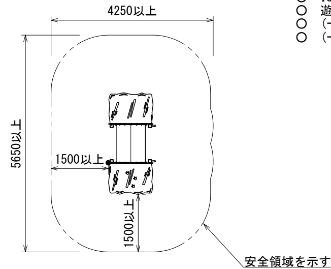
安全領域図 S=1:100
