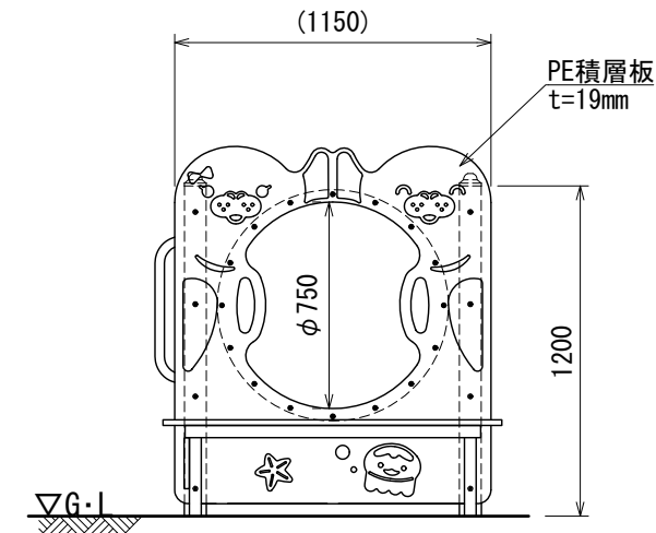
背面図
