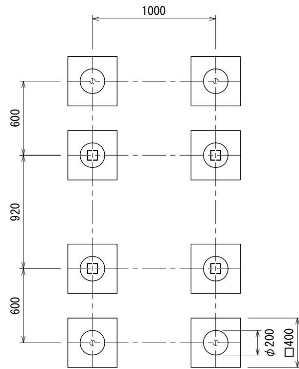
基礎伏図
