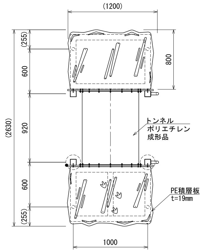
平面図
