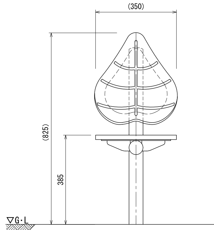
立面図
