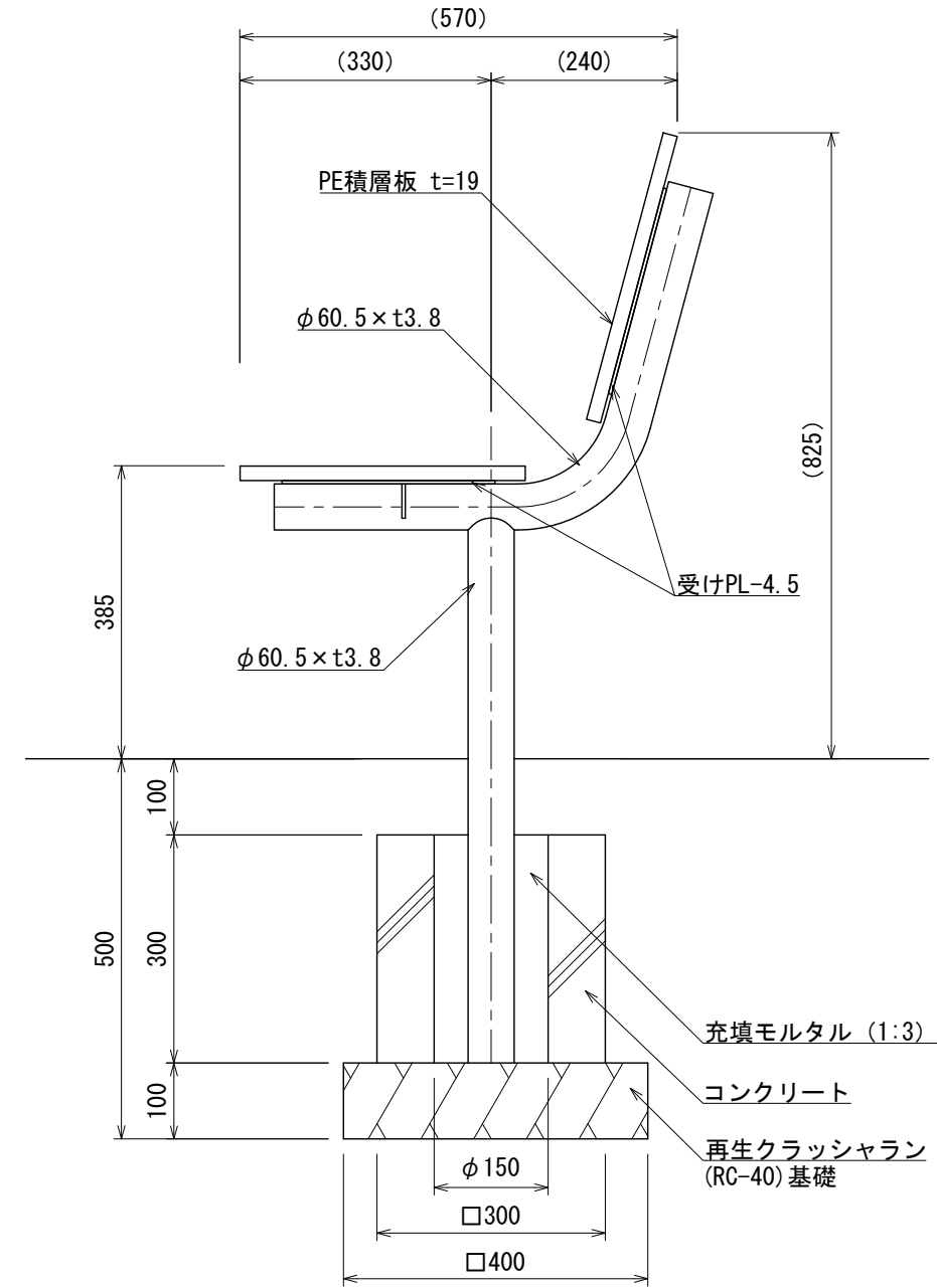
断面図
