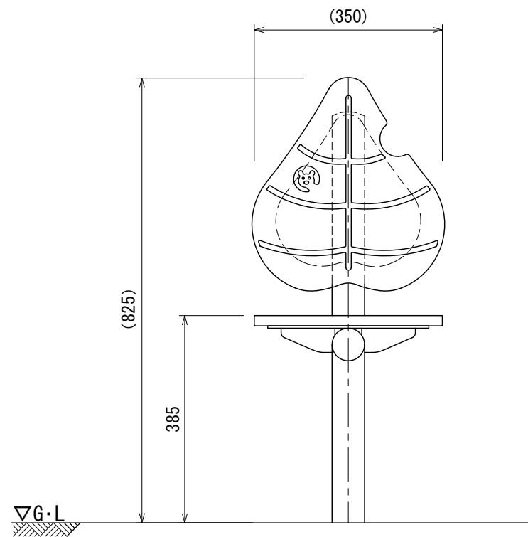
立面図
