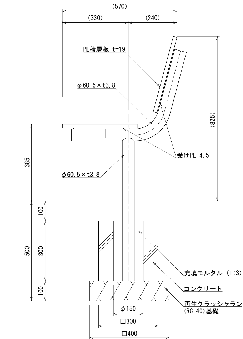
断面図
