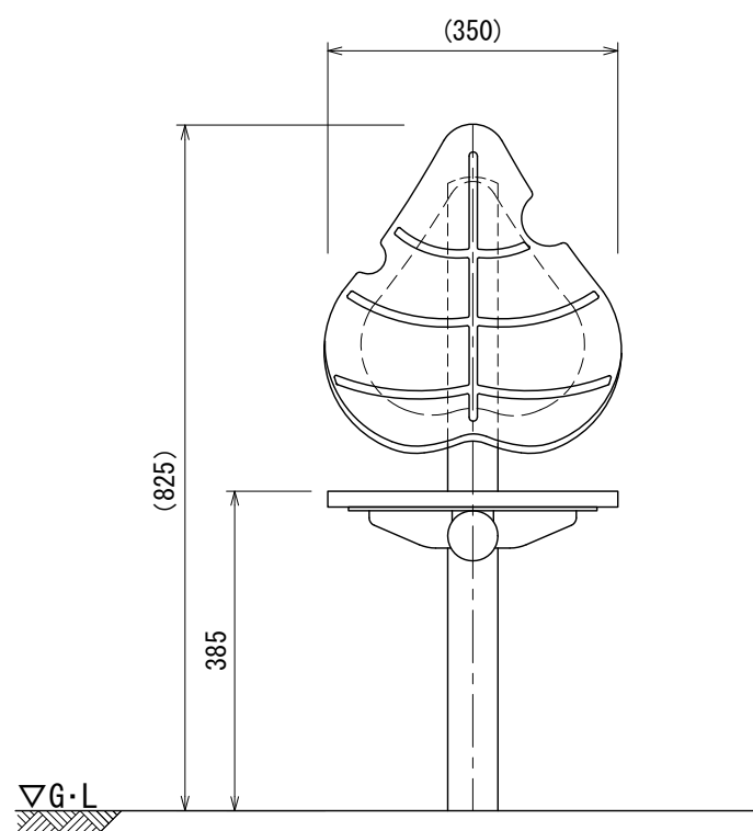
立面図
