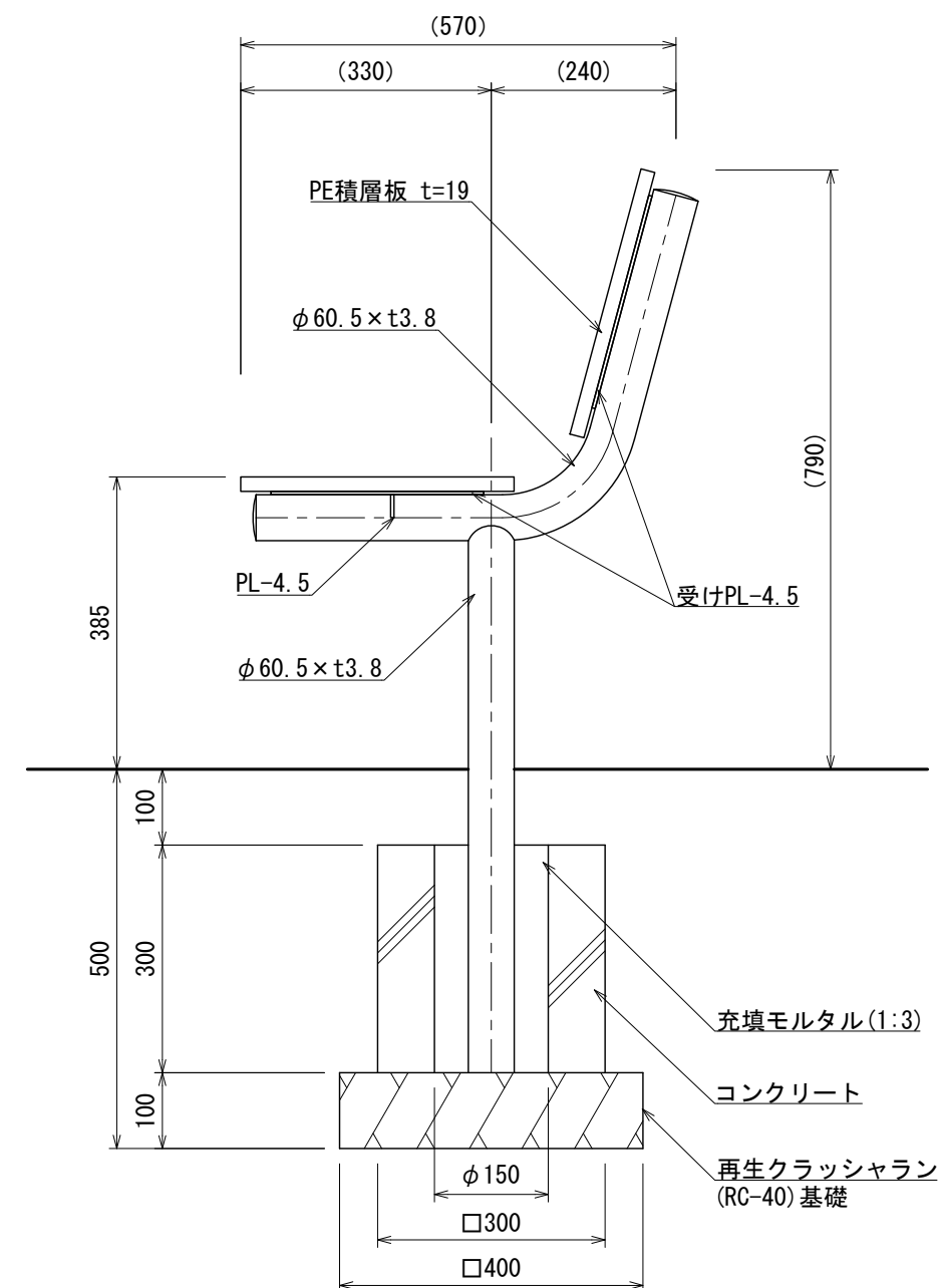
断面図
