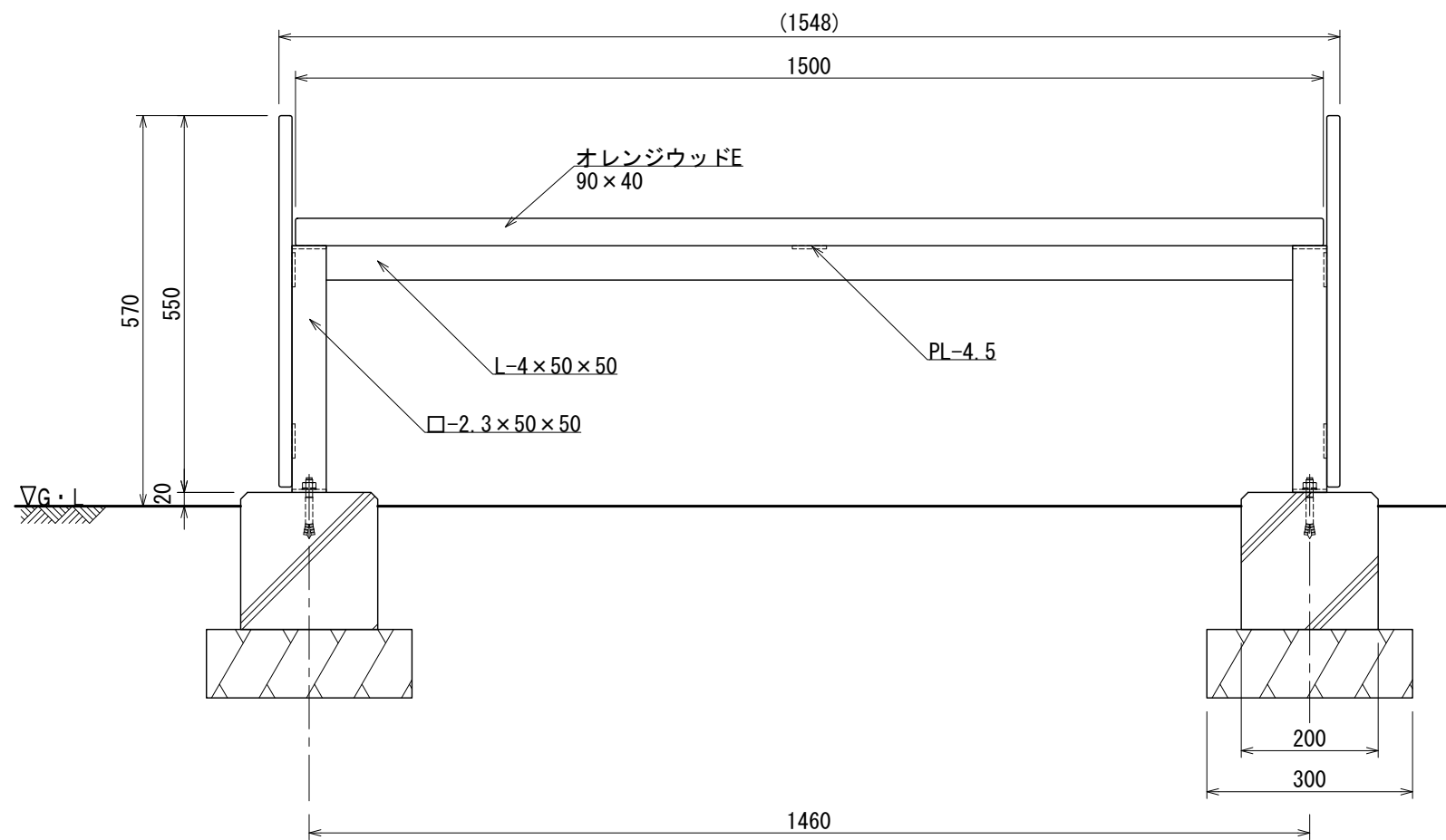
〔座部断面図(2層構造)〕
