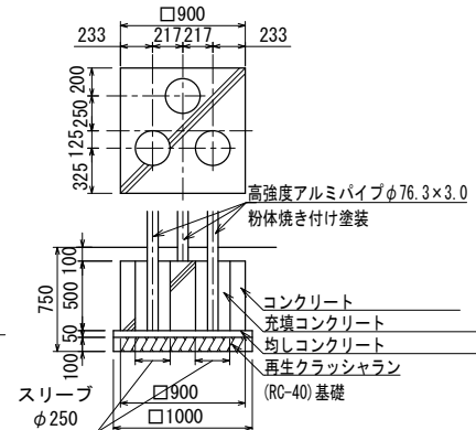
E' 基礎詳細図 (スリーブ穴位置や方向に注意する事)
